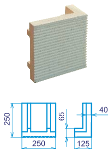
AK-RV010 - Roh římsový 500x250x125x 40 - 6,96kg
