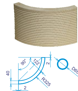
AK-OA325 - Oblouk R325 8,98kg
