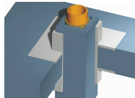
Keramické komíny
