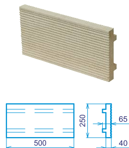
AK-DV010 - Deska římsová 500x250x40 - 10,46kg
