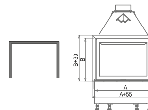
RÁM 3S třístranný
