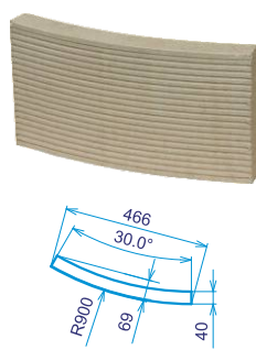
AK-OA900 - Oblouk R900 9,4kg
